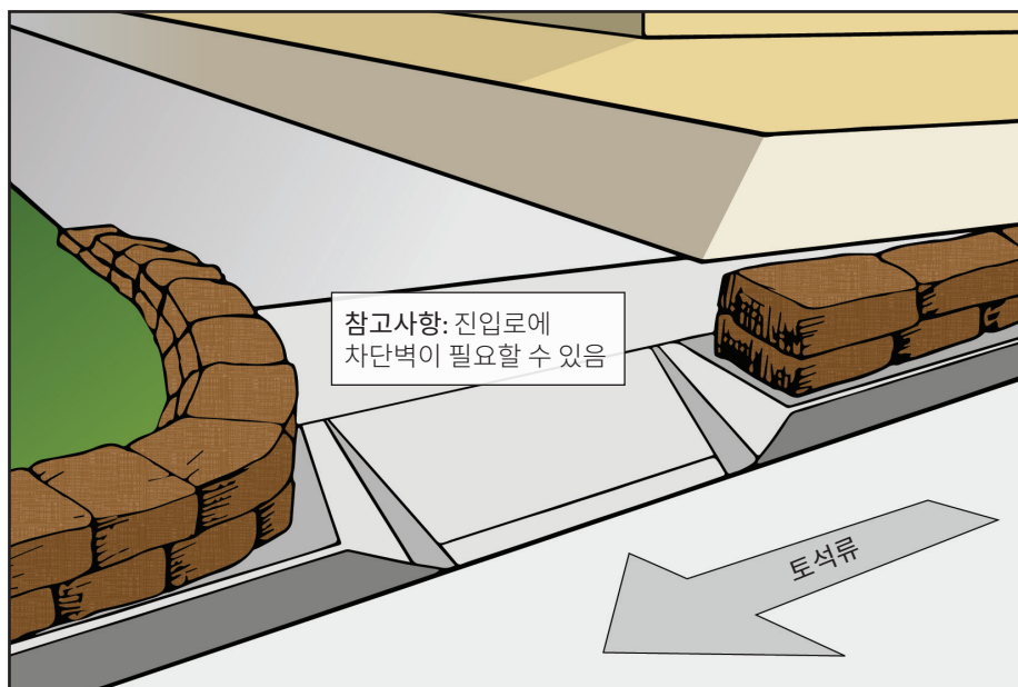
그림 8 - 도로의 토석류 또는 폭우 유출수 차단
